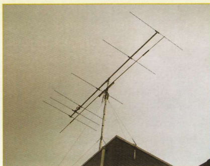
Een enkel element voor HF, met daarboven een 6 meter-antenne. Hier zal de invloed op de afstemming van de HF-antenne van de boom van de yagi goed merkbaar zijn. Andersom zal de invloed daarentegen nihil zijn.
